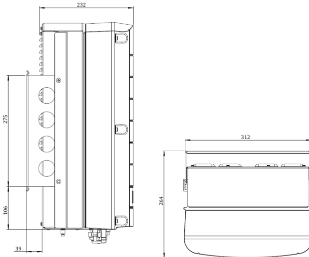
Abbildung 30: Dreiphasenwechselrichter mit Halterung - Seitenansicht und Draufsicht
