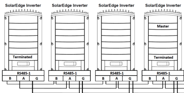
Abbildung 22: Anschluss der Wechselrichter in einem Bus
