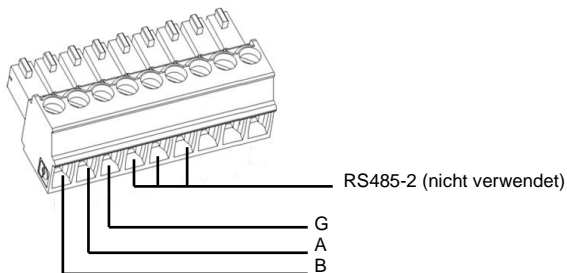
Abbildung 21: RS485-/RS232-Klemmleiste
