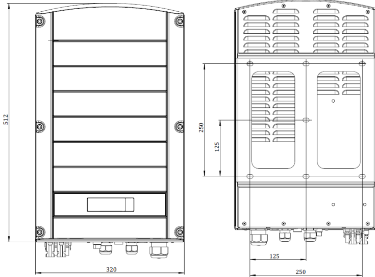
Abbildung 29: Dreiphasenwechselrichter mit Halterung - Vorder- und Rückansicht
