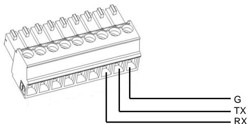
Abbildung 25: RS485/RS232-Klemmleiste
