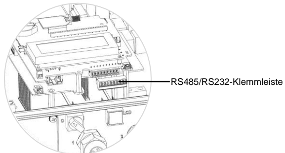
Abbildung 24: RS485/RS232 9-polige Klemmleiste
