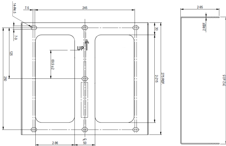
Abbildung 31: Montagehalterung des Dreiphasenwechselrichters
