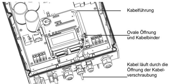
Abbildung 37 – Kabelführung des Steuerkabels für die Leistungsreduzierung
