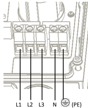
Abbildung 10: Dreiphasiger Wechselrichter - AC-Klemmleisten:
