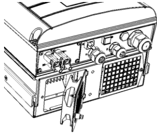
Abbildung 32: Wechselrichter Lüfter 2
