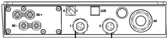
Abbildung 14: Kommunikationsverschraubungen
