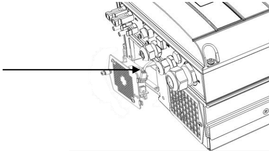
Abbildung 33: Lüfteranschluss
