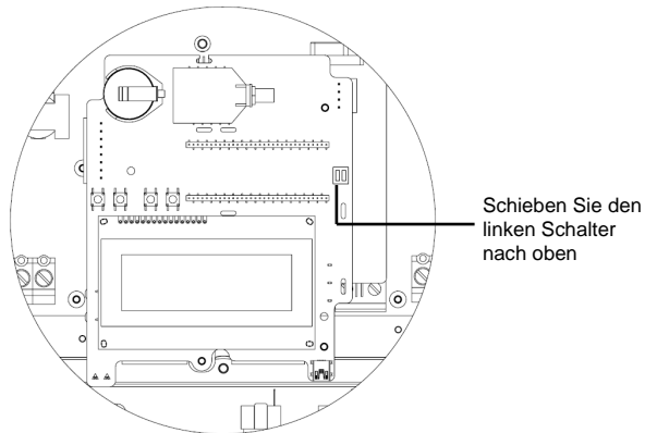
Abbildung 23: RS485 DIP-Schalter
