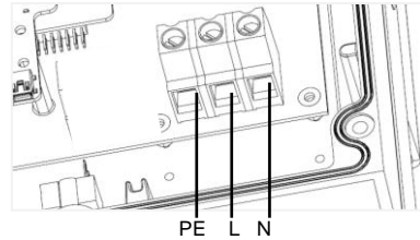
Abbildung 9: Einphasiger Wechselrichter - AC-Klemmleisten
