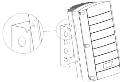
Abbildung 6: Einhängen des Wechselrichters in der Halterung
