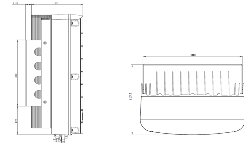
Abbildung 27: Einphasenwechselrichter mit Halterung – Seitenansicht und Draufsicht
