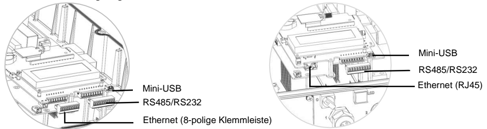
Abbildung 15: Interne Anschlüsse
