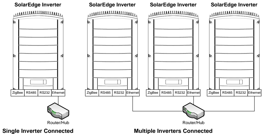
Abbildung 16: Beispiel einer Ethernet-Verbindung
