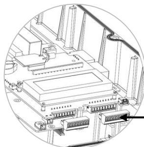
Abbildung 20: Die RS485-/RS232-Klemmleiste
