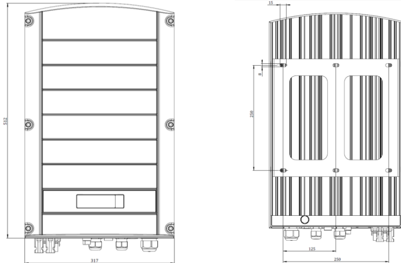
Abbildung 26: Einphasenwechselrichter mit Halterung - Vorder- und Rückansicht
