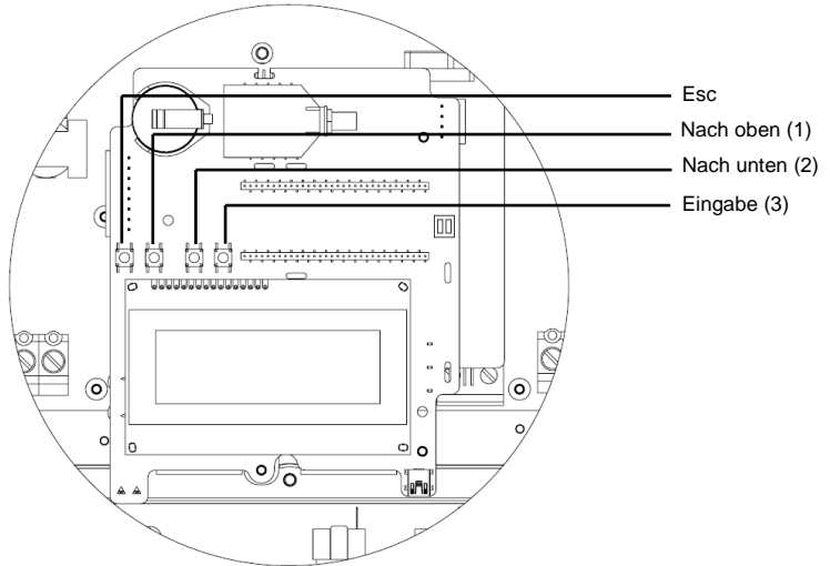
Abbildung 13: Interne LCD Bedientasten
