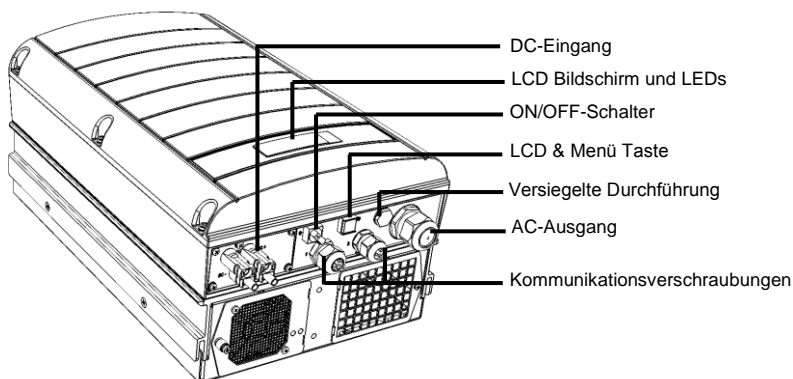
Abbildung 3: Wechselrichteranschlüsse (Beispiel: Dreiphasen-Gerät)
