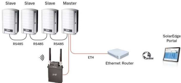
Abbildung 38 – FRSE-Anschluss in einer Umgebung mit mehreren Wechselrichtern
