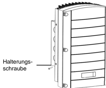
Abbildung 7: Einführen der Schrauben in die äußeren Rippen des Kühlkörpers
