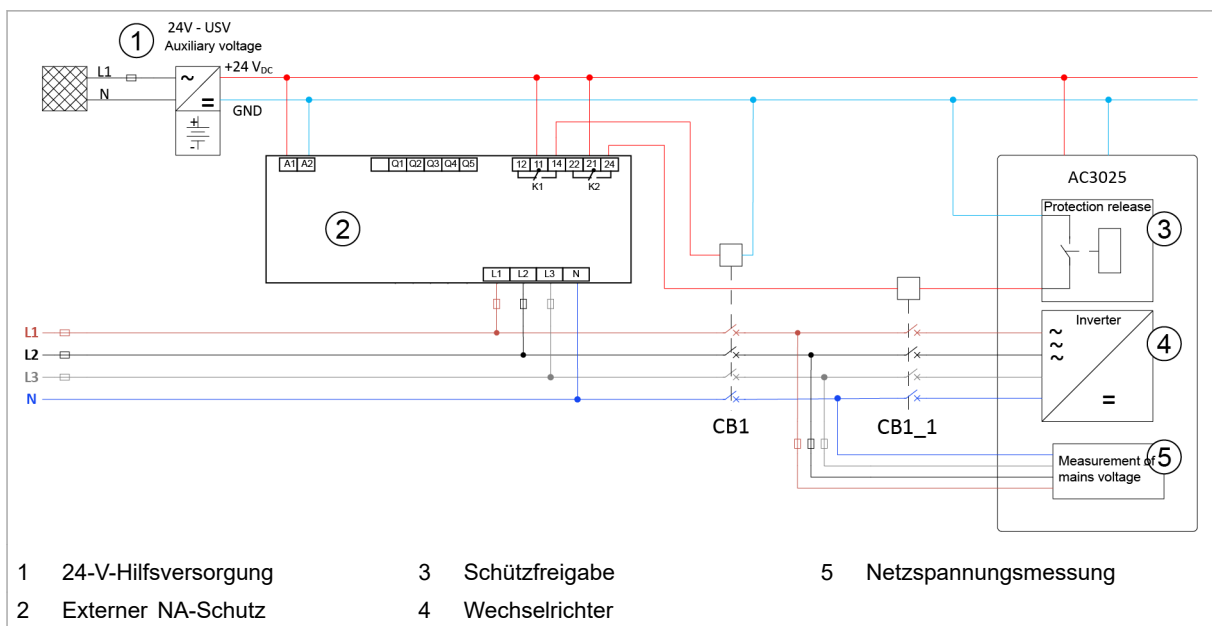
Beispiel zur Einbindung von Eigen- und Entkupplungsschutz
