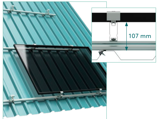
Landscape-Ausrichtung mit Eindreh-Profil Pro70 und Modulträgerprofil Pro35
