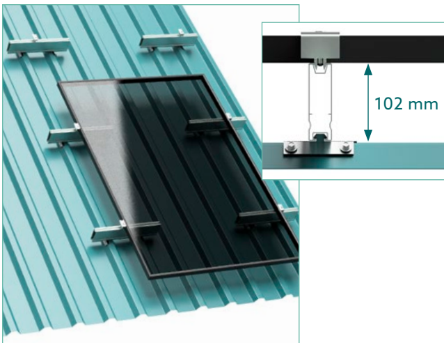
Portrait-Ausrichtung mit Montageträgerprofil Pro100
