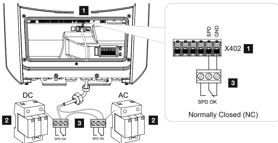
Abb. 5: Überspannungsschutz (SPD) als Öffner
