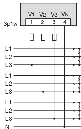
Abb.: Spannungsmessung in bis zu drei symmetrisch belasteten Dreiphasen-Dreileitersystemen
