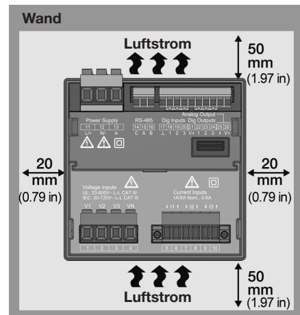
Abb. Einbaulage des UMG 96-PAJ-MID+ (Rückansicht)
