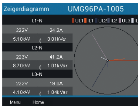
Abb. Zeigerdiagramm
