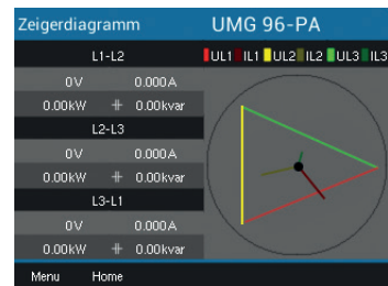
Anzeige von Spannungsverlauf von L1-L2, L2-L3, L3-L1
