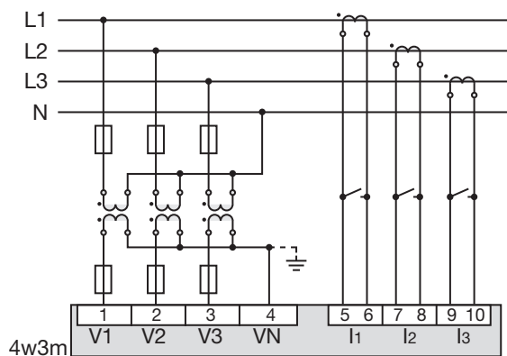
Abb. Anschlussvariante 4w3m hv - Messung über 3 Spannungswandler in einem Dreiphasen-4-Leiternetz mit unsymmetrischer Belastung.
