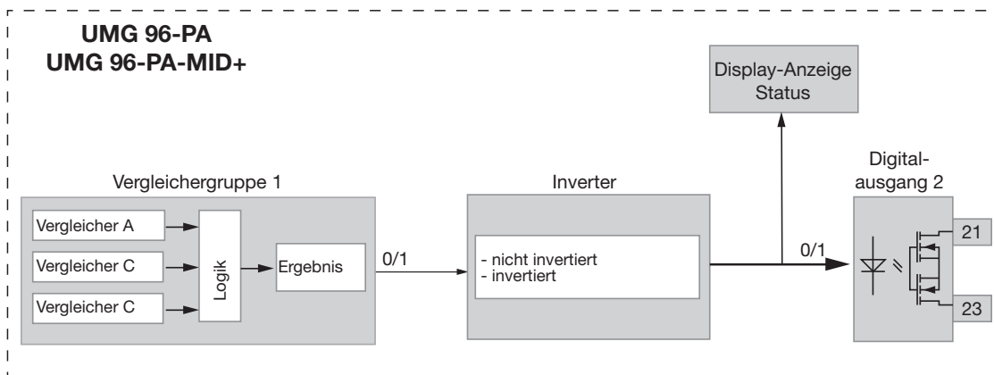
Abb. Blockschaltbild "Verwendung des Digitalausgangs 2 zur Grenzwertüberwachung"
