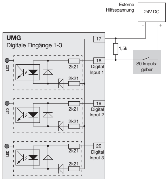
Abb. Beispiel für den Anschluss eines S0 Impulsgebers an digitalen Eingang 1.
