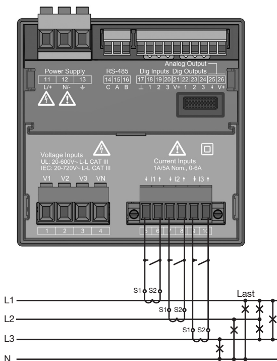
Abb. Anschlussbeispiel „Strommessung über Stromwandler“.
