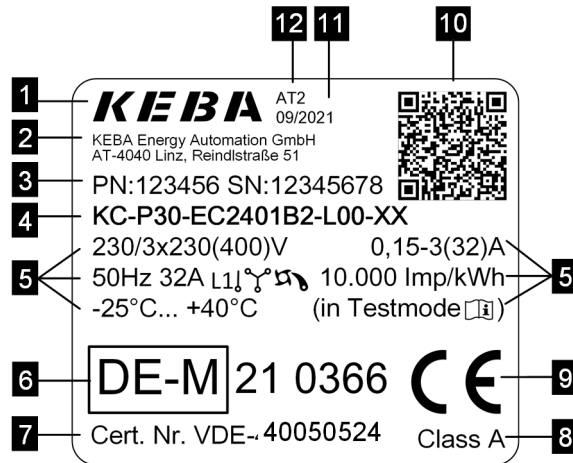
Abb. 3-2: Typenschild (Beispiel)
