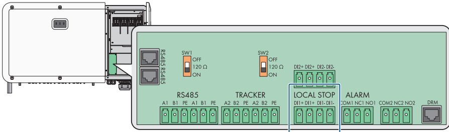
Abbildung 10: Digitale Eingänge für die Schnell-Stopp-Funktion auf der COM-Baugruppe
