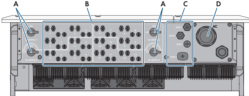
Abbildung 7: Gehäuseöffnungen an der Unterseite des Wechselrichters
