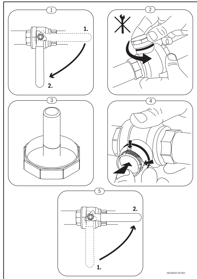
Bild 14 Siebreinigung
