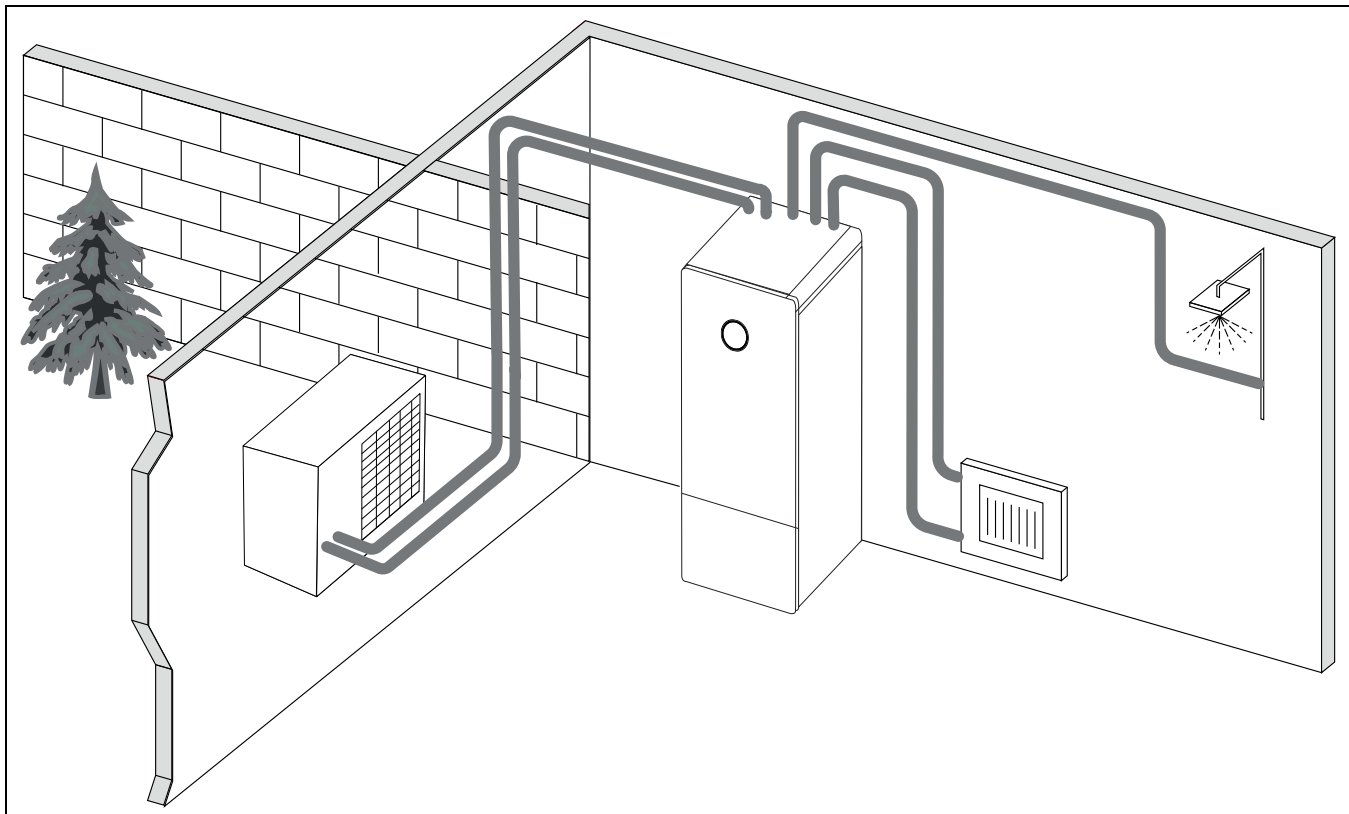
Bild 7 Wärmepumpe AW OR, Inneneinheit Compress 5800/6800i 12 M mit integriertem Warmwasserspeicher und elektrischem Zuheizter
