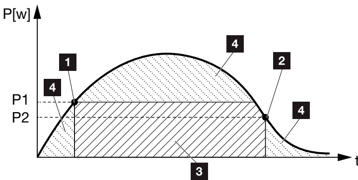
Abb. 66: Kurve Eigenverbrauch (Funktion 2)
