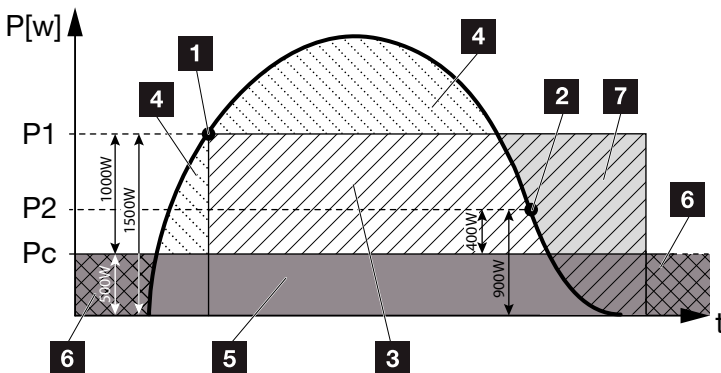
Abb. 67: Kurve Dynamischer Eigenverbrauch (Funktion 2)
