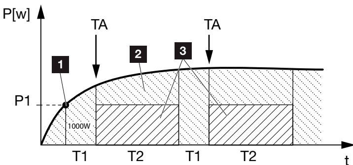
Abb. 64: Kurve Eigenverbrauch (Funktion 1)
