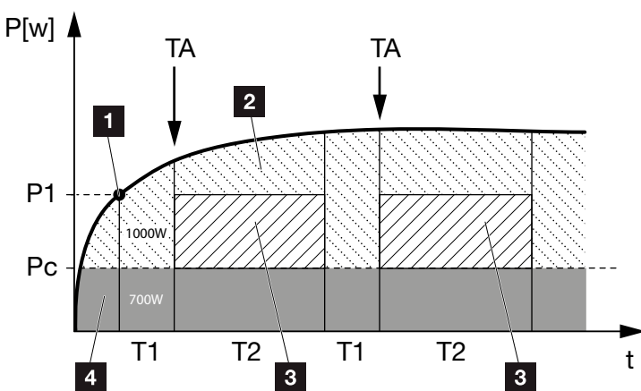
Abb. 65: Kurve Dynamischer Eigenverbrauch (Funktion 1) Leistungsgrenze
