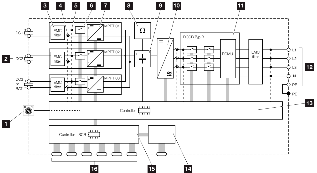
Abb. 75: Blockschaltbild
