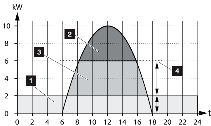
Abb. 57: Regelung mit intelligenter Batteriesteuerung
