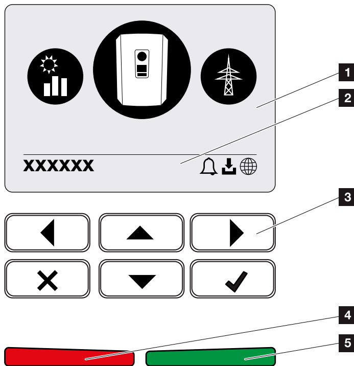
Abb. 13: Bedienfeld
