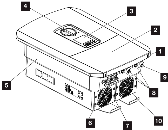
Abb. 9: Wechselrichter (Außenansicht)
