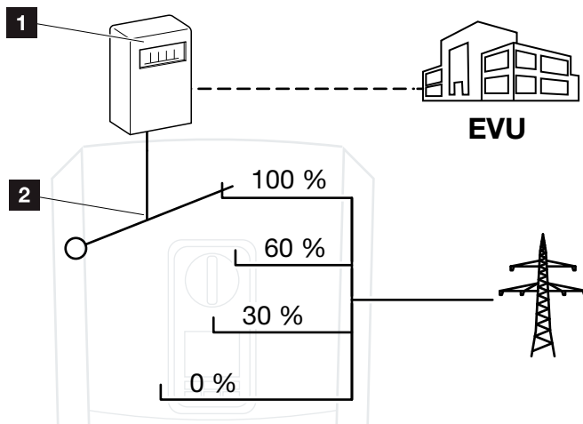
Abb. 59: Wirkleistungssteuerung mit Rundsteuerempfänger
