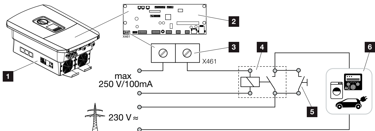
Abb. 32: Anschluss Eigenverbraucher
