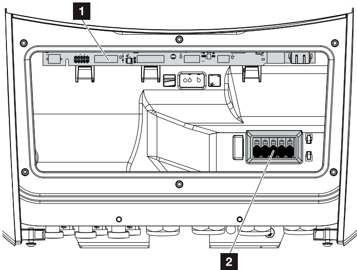
Abb. 12: Wechselrichter (Innenansicht)
