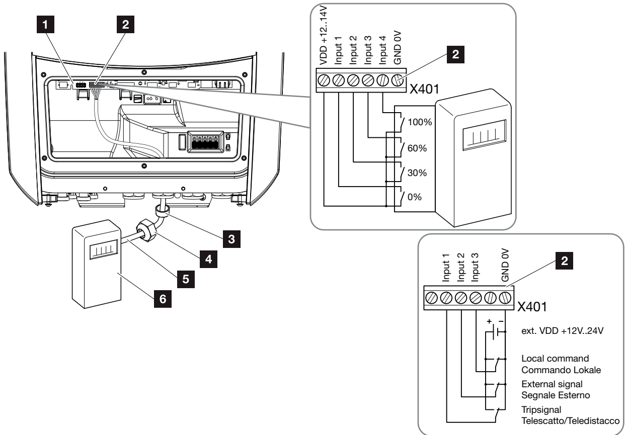
Abb. 31: Anschluss Rundsteuerempfänger !
