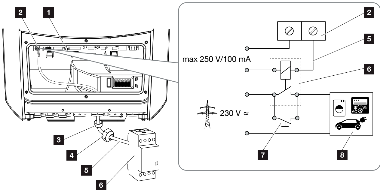
Abb. 62: Elektrischer Anschluss Eigenverbrauch
