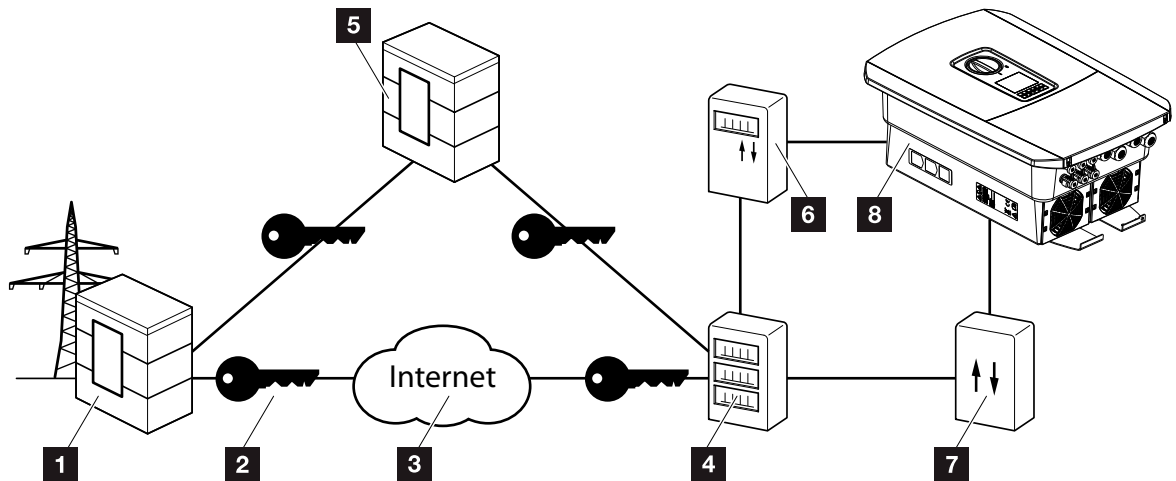
Abb. 60: Anschluss Intelligente Messsysteme
