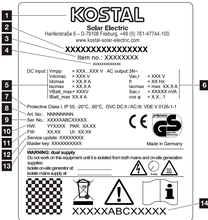
Abb. 76: Typenschild
