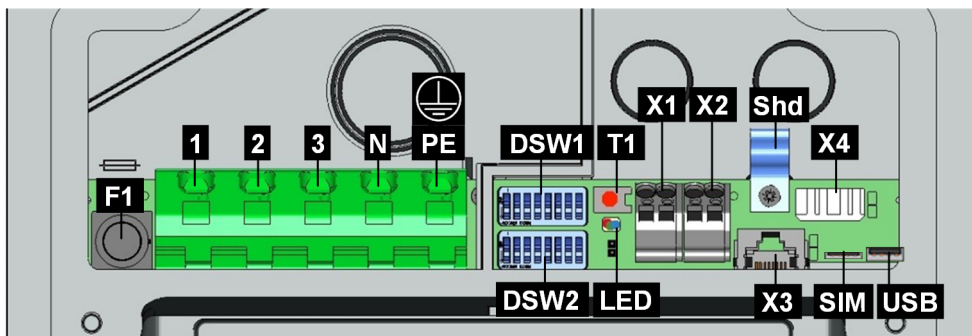
Abb. 7-16: Anschlussübersicht
