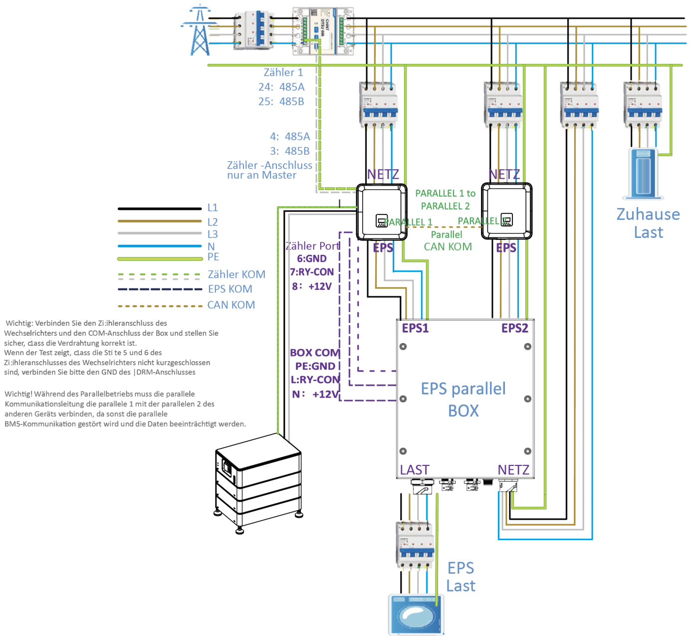
Systemdiagramm von zwei H3 offline und parallel
