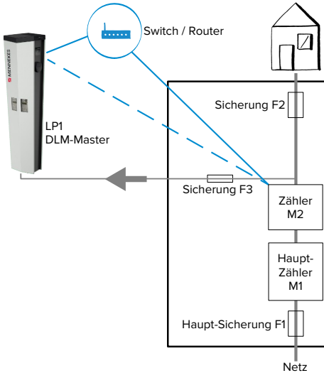
Abb. 18: Energiezähler misst externe Verbraucher und Ladestation (Gesamtverbrauch)
