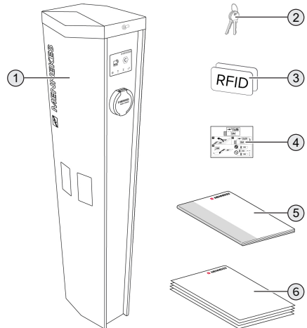
Abb. 2: Lieferumfang
