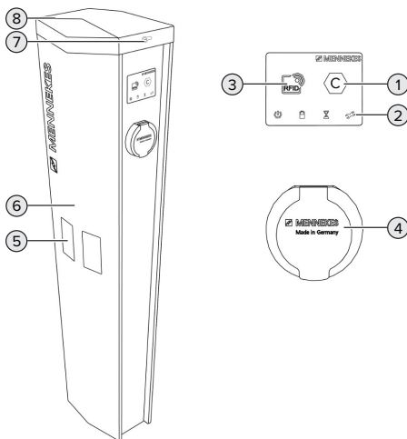
Abb. 3: Außenansicht
