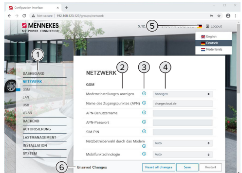
Abb. 16: Aufbau Weboberfläche bei Firmware Version 5.12.3 (Beispiel)
