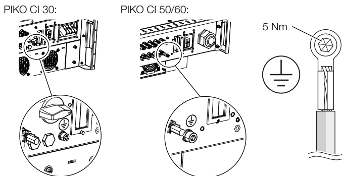
Abb. 18: Länderspezifischer PE-Anschluss außen
