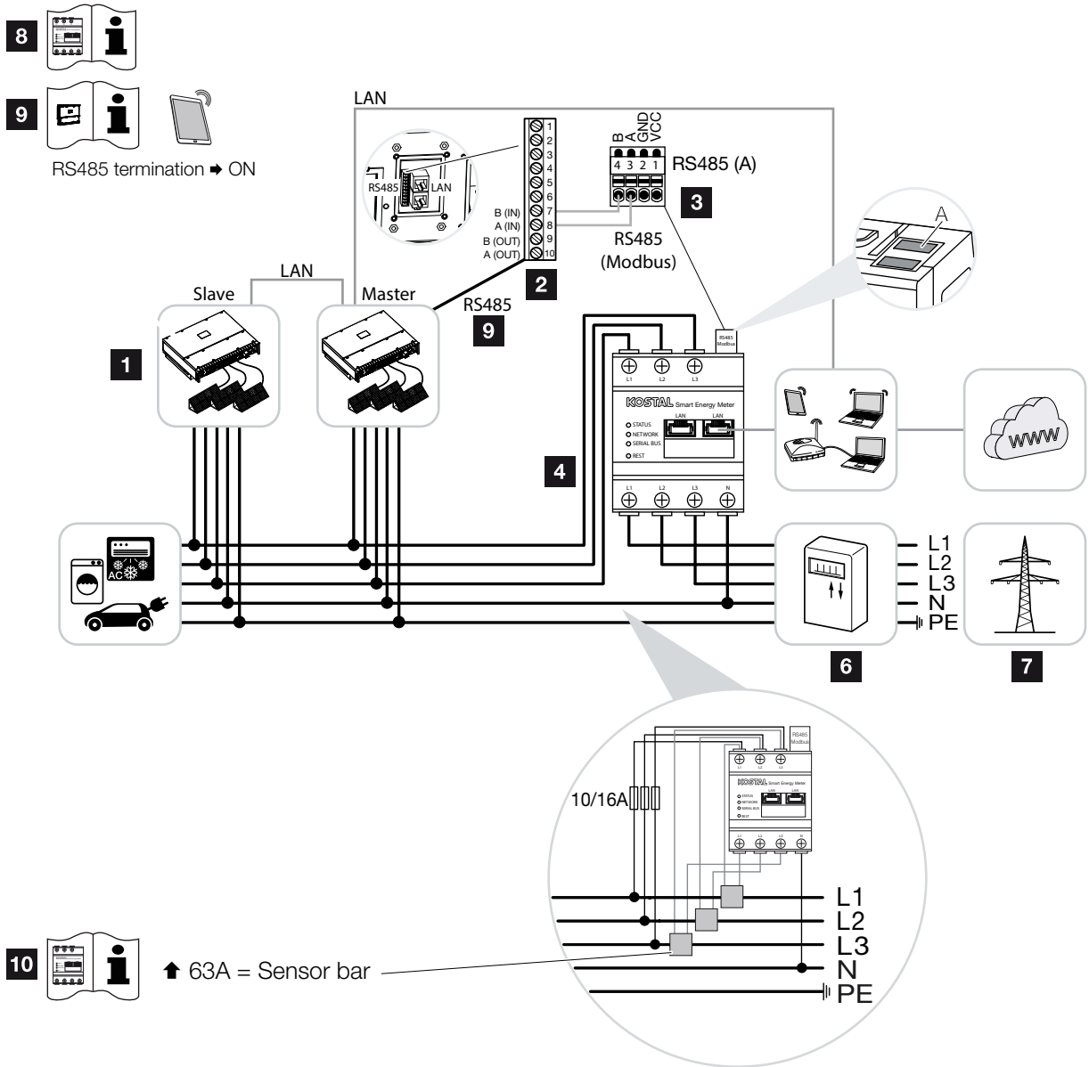
Abb. 25: Anschlussplan Energiezähler - Netzanschluss
