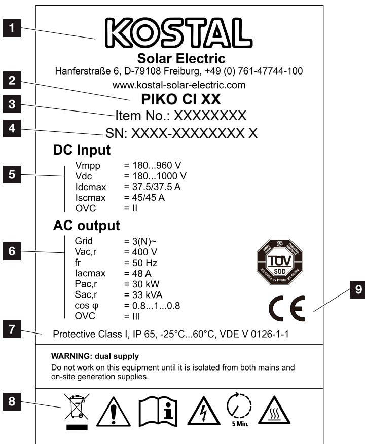
Abb. 37: Typenschild
