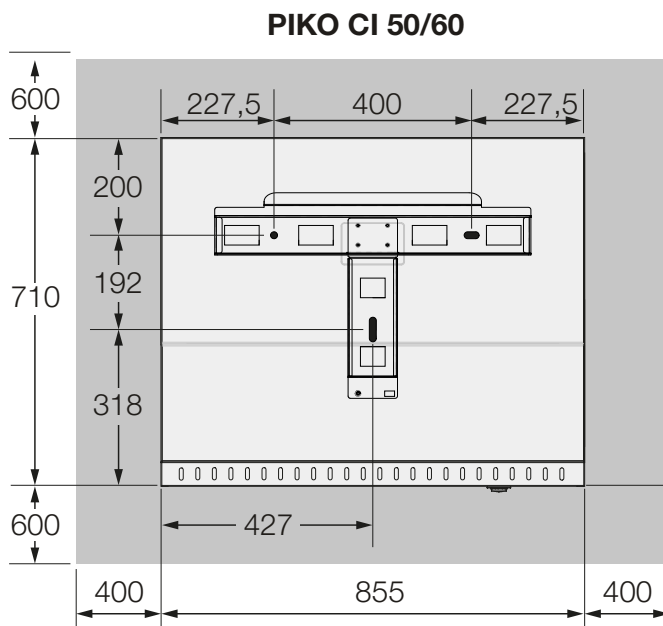
Abb. 12: Montagemaße mit Halterung
