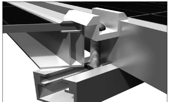
Beispiel 1 – Klemmflügel
